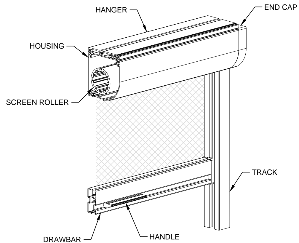
SMART SCREEN SCALE: 3" = 1'-0"
