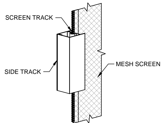
DETAIL 1 SCALE: 3" = 1'-0"
