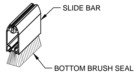
DETAIL 2 SCALE: 3" = 1'-0"
